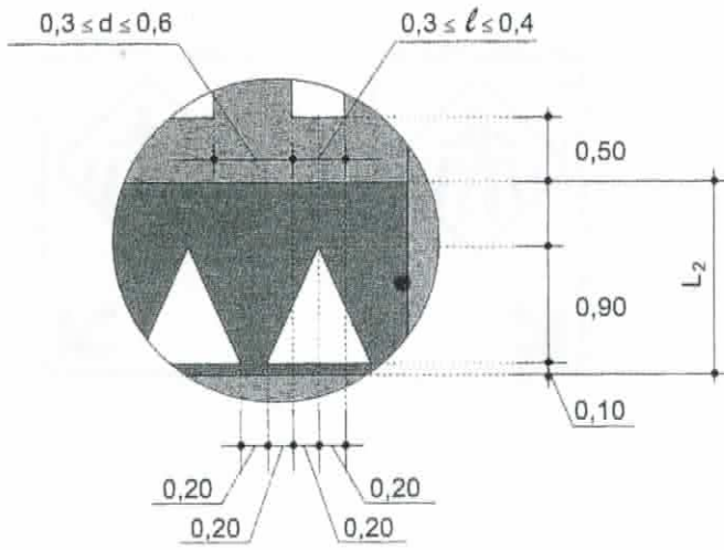
DETALHE A
