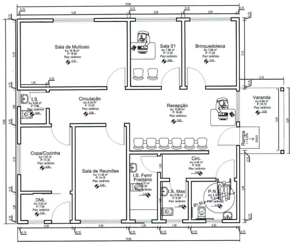
Planta Baixa Esc. 1/100 Área: 114,78 m²
