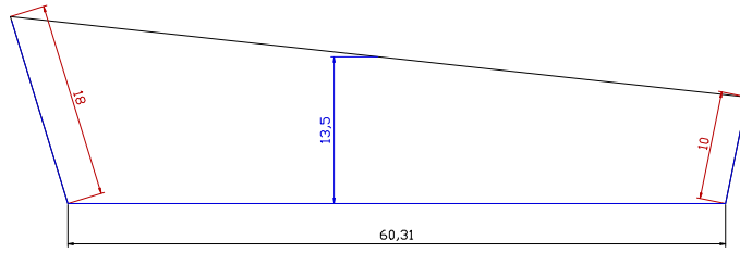
PERFIL ESQUEMÁTICO DA AMPLIAÇÃO DO ATERRO
